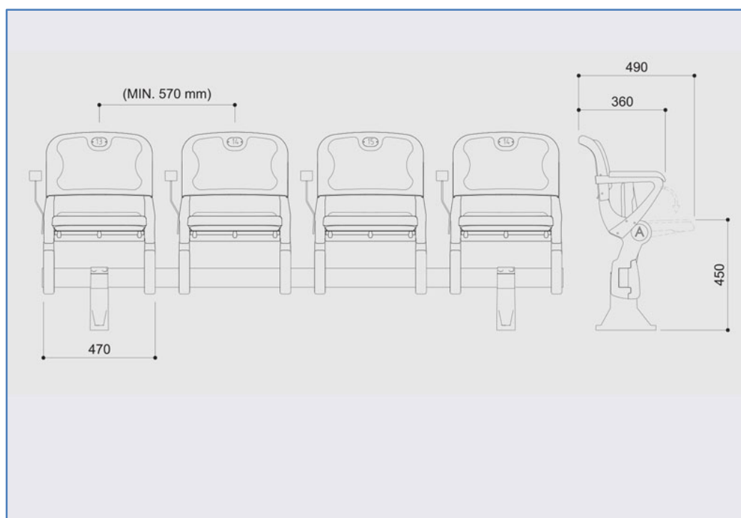
Στήριξη στο έδαφος με μπράτσα
