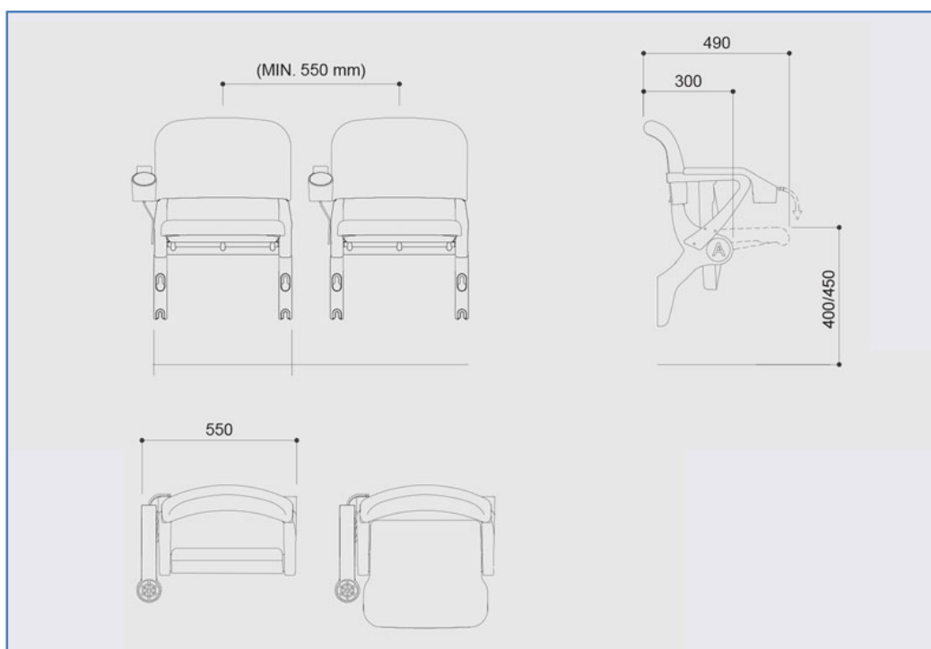
Στήριξη στο ρίχτι, με μπράτσα με ποτηροθήκη
