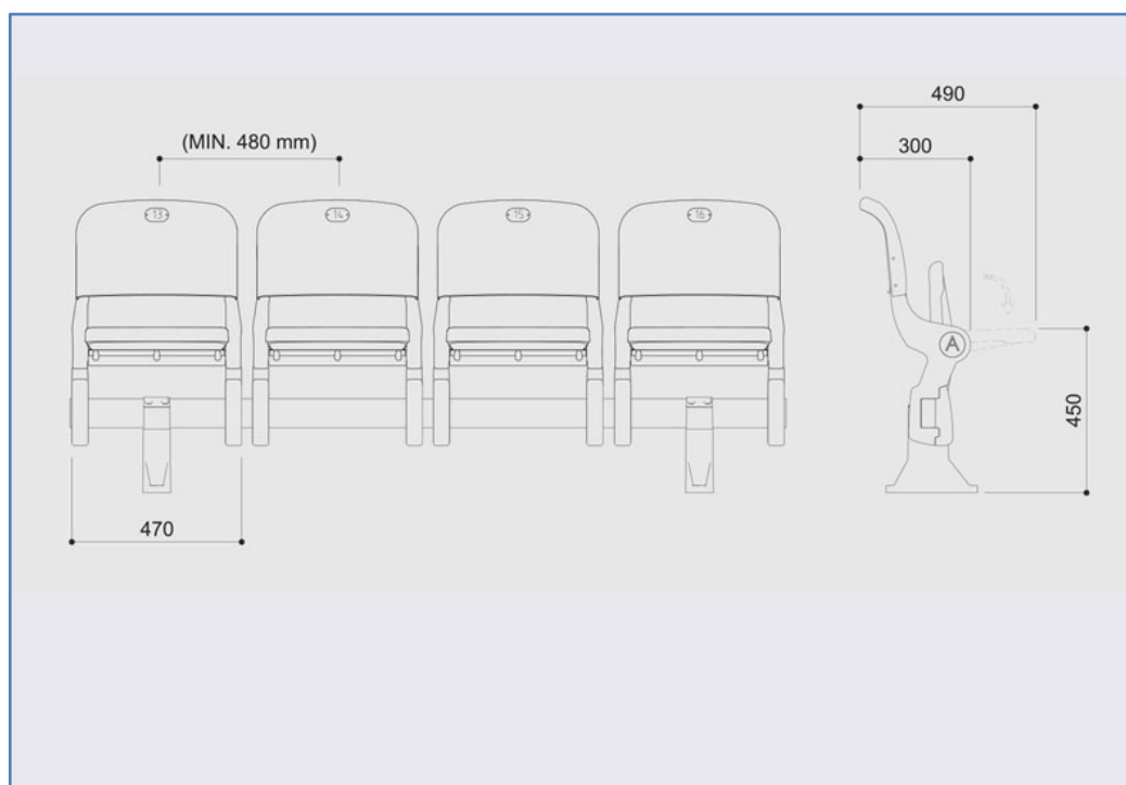
Στήριξη στο έδαφος χωρίς μπράτσα
