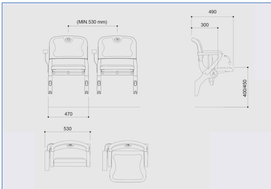
Στήριξη στο ρίχτι, με μπράτσα
