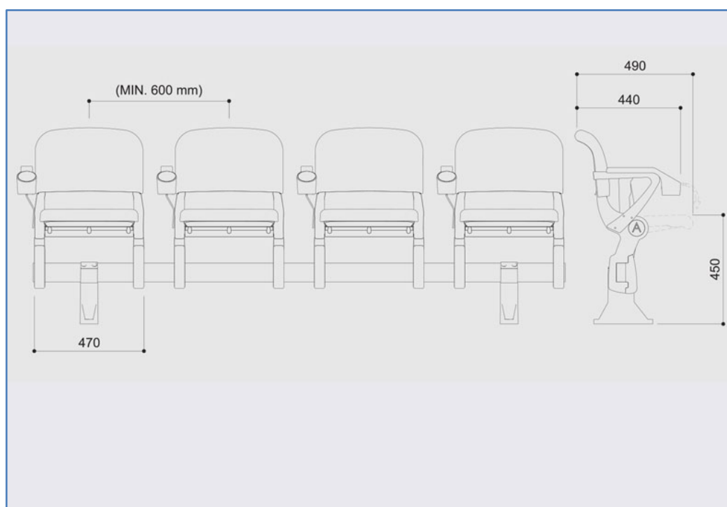
Στήριξη στο έδαφος, με μπράτσα και ποτηροθήκη
