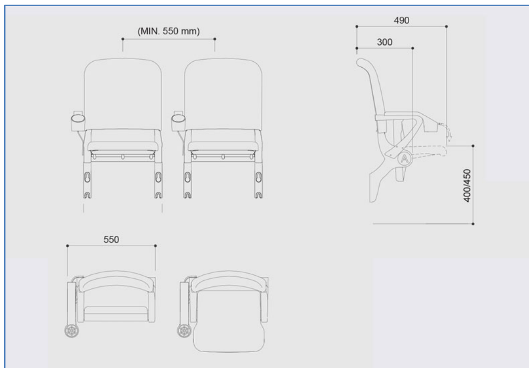
Στήριξη στο ρίχτι, ψηλή πλάτη με ύφασμα και μπράτσα με ποτηροθήκη
